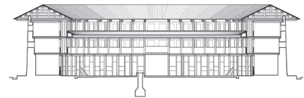
Fig. 2 - Architettura di terra: la costruzione della forma. Chungui Lou | Hekeng, Nanjing, Fujian, Cina. A sinistra: pianta, prospetto, sezione. A destra: sezione costruttiva, assonometria.
