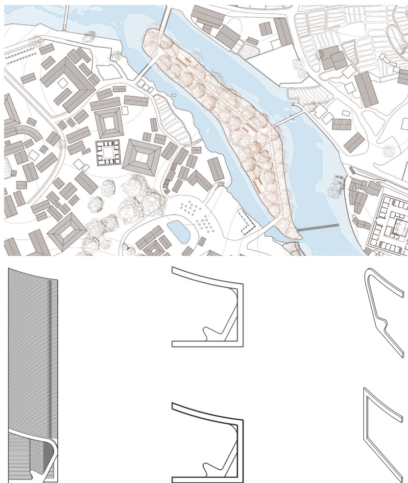
Fig. 7 - In alto: masterplan area 3. Stare: la zona d'ombra. In basso: pianta, prospetto, sezione, assonometrie della zona d'ombra.
